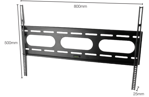
Ref. 903130 Support écran plasma 37-60"
